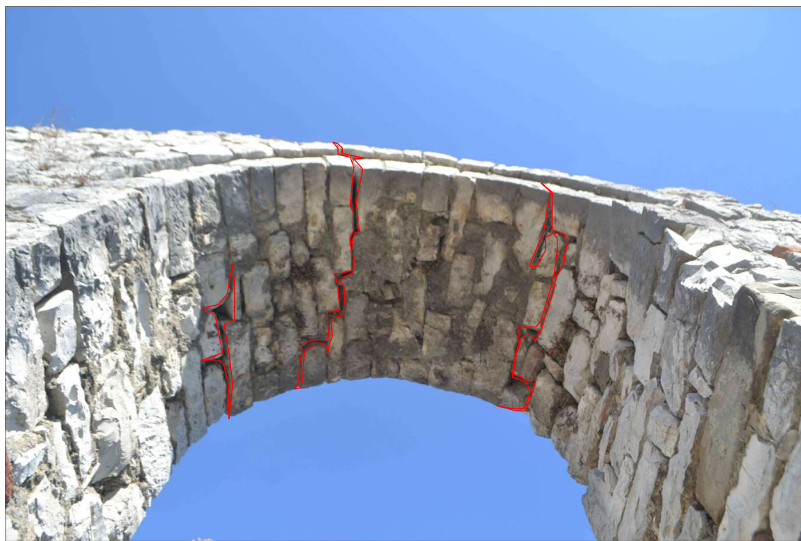
Fig. 78: Çedim dhe dëmtim i harkut prej guri të hyrjes së anës jugore në kullën Nr.1. Foto: Dritan Çoku, 30.08.2021, DRTK-Berat.
