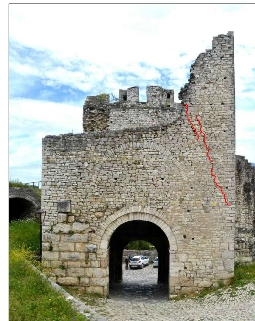
Fig. 73: Kulla Nr. 24 (faqja e brendshme) - Gjendja ekzistuese. Foto: Dritan Çoku, 28.07.2021, DRTK-Berat.
