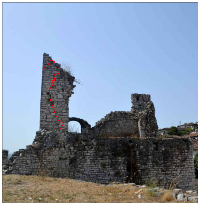
Fig. 72: Krisje vertikale në qoshen verilindore të kullës Nr.24, e cila rrezikon shkëputjen e qoshes së sipërme të murit (Pamja veriore e kullës Nr. 24). Foto: Dritan Çoku, dt.17.05.2021, DRTK-Berat.
