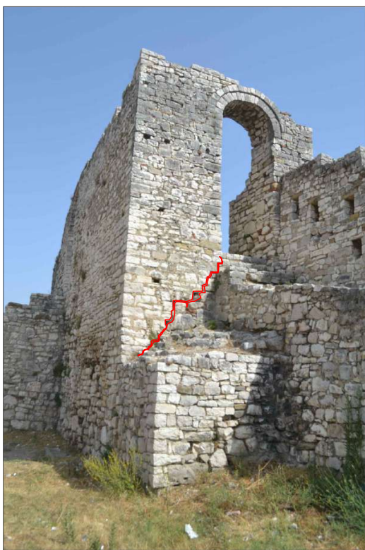
Fig. 77: Çarje e muraturës së gurit nga fundi i hyrjes për në kullën Nr.1 e deri në pjesën e poshtme të qoshes jugperëndimore të kullës. Foto: Dritan Çoku, 28.07.2021, DRTK-Berat.
